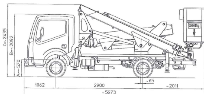
DIMENSIONS
